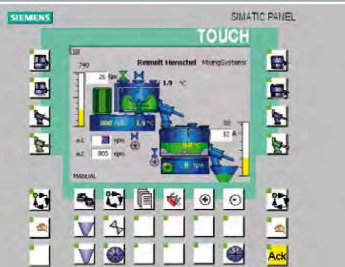
S7 und Visualisierung mit Bedienpanel S7 and visualisation with operator panel
